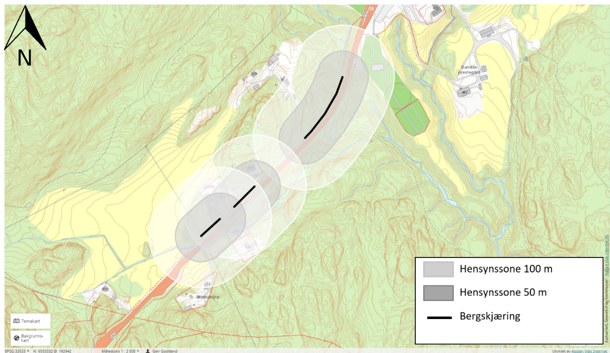
Figur 87: Omtrentlig hensynssone for sprengningsarbeid ved profilnummer 290-450, 550-620 og 670-710.
