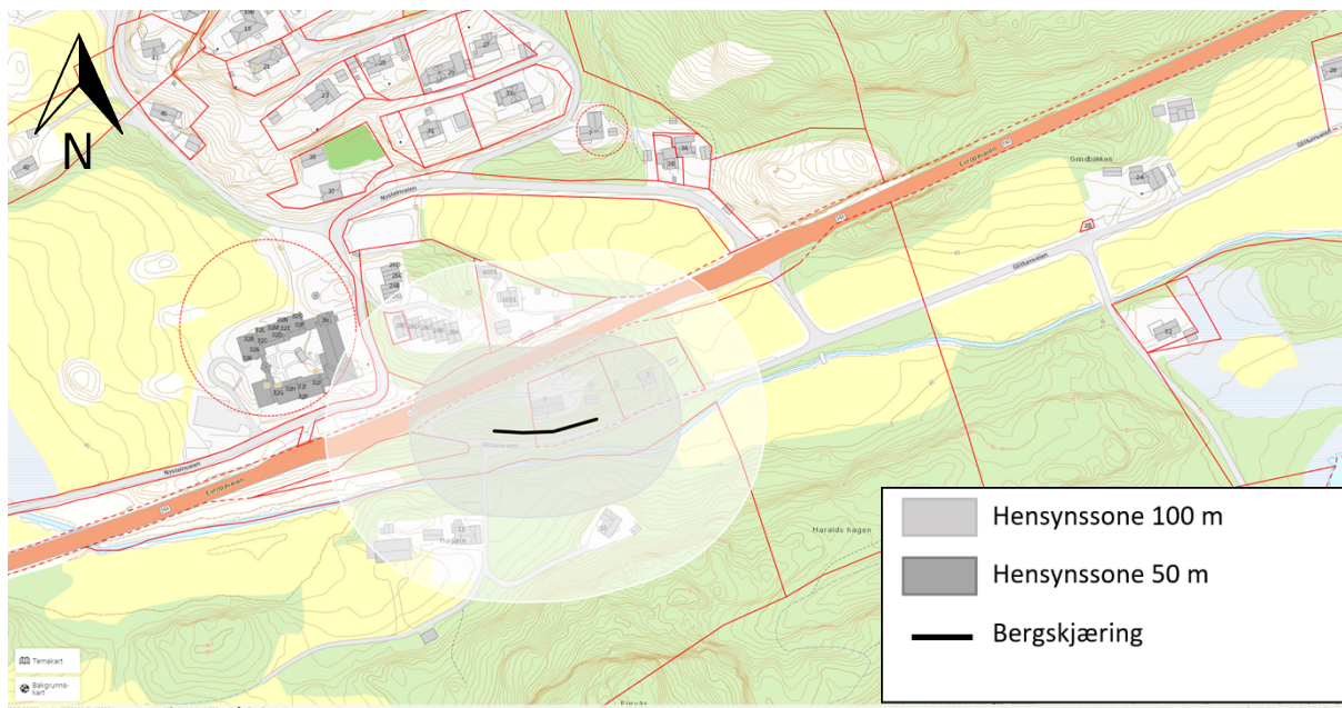
Figur 91: Omtrentlig hensynssone for sprengningsarbeid ved profilnummer 2280-2320.
