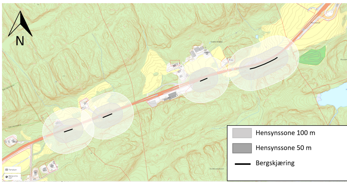
Figur 90: Omtrentlig hensynssone for sprengningsarbeid ved profilnummer 160-270, 535-545, 930-970 og 1130-1160.
