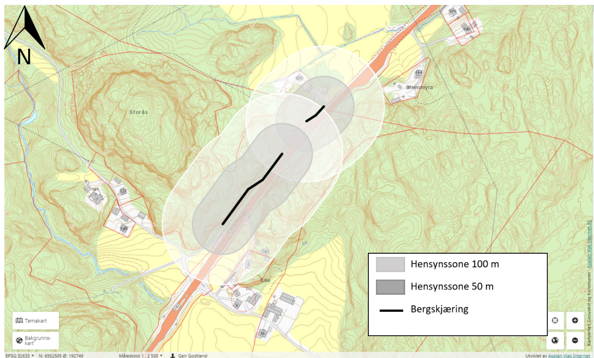
Figur 88: Omtrentlig hensynssone for sprengningsarbeid ved profilnummer 920-960 og 1010-1180.
