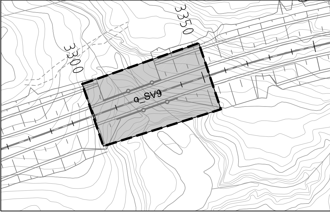
Vertikalnivå 3 - Søtholtbekkbrua
