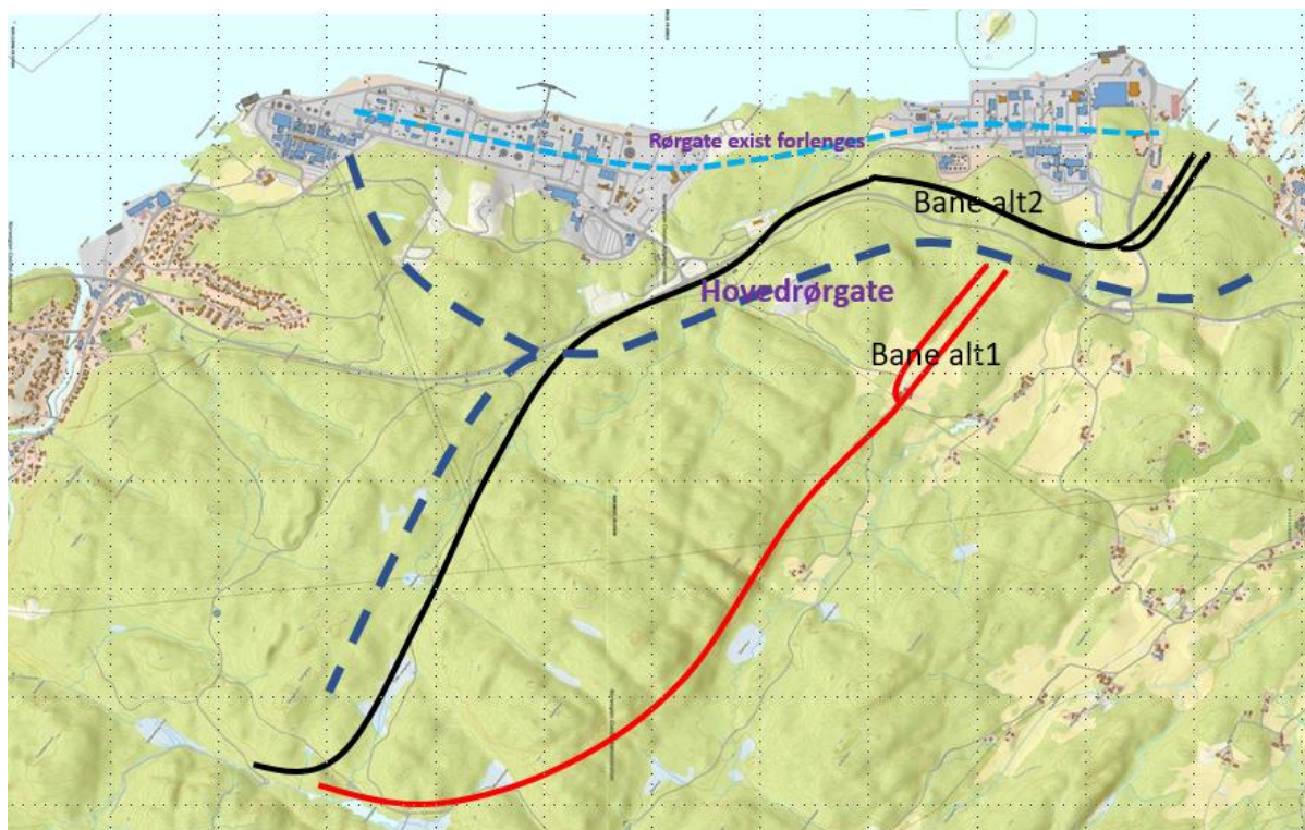
Figur 6-29 Skisse som vise mulig påkopling av sidespor til Grenlandsbanen og etablering av terminalområde
