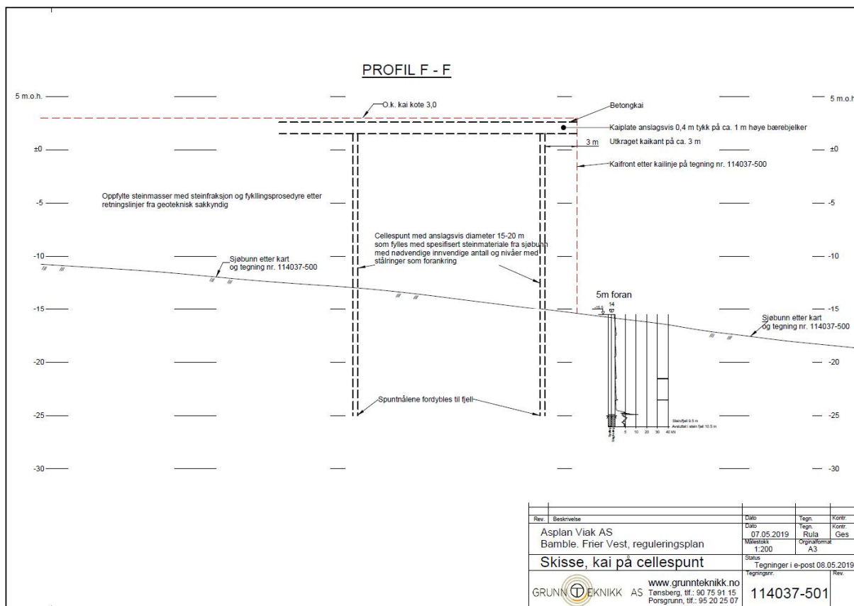
Figur 6-33 Front etableres med cellespunt. Tegning nr. 114037-501
