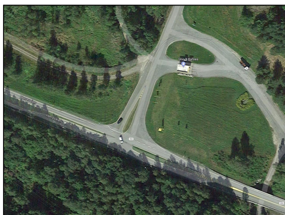
Figur 3-16 Avkjøring til Rafnes. Kanalisert kryss mellom fv. 353 og avkjøring til Rafnes industriområde. 35 m langt venstresvingefelt fra nordvest. (google.com/maps, 21.02.2019)
