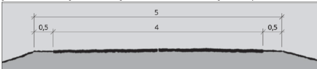
Figur 50: Tverrprofil A1, 5 m vegbredde (mål i m). Kilde: SVV HB100 Veg- og gateutforming.
