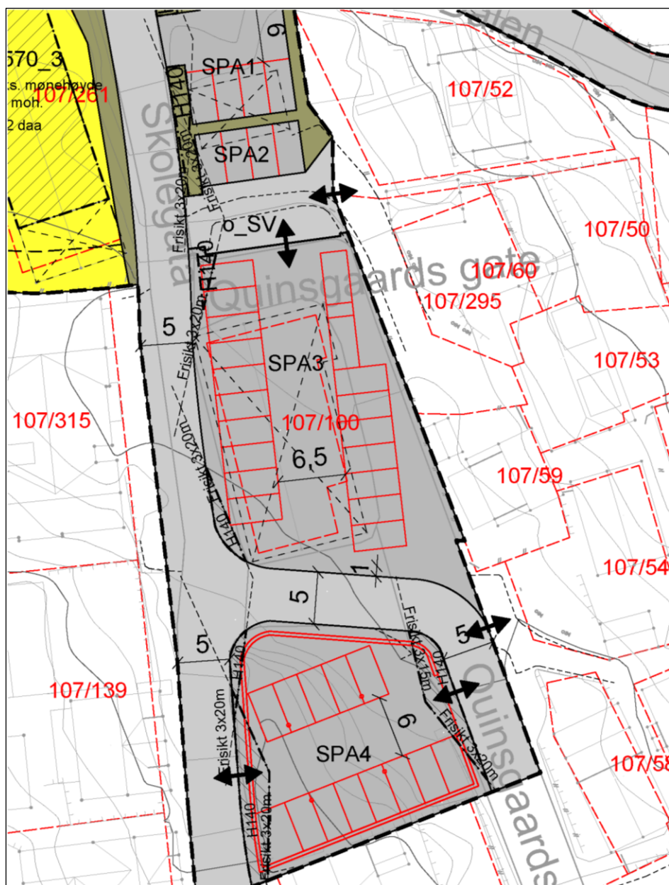
Figur 48: Utsnitt av forslag til reguleringsplan for nye parkeringsplasser SPA1, SPA2, SPA3 og SPA4.
