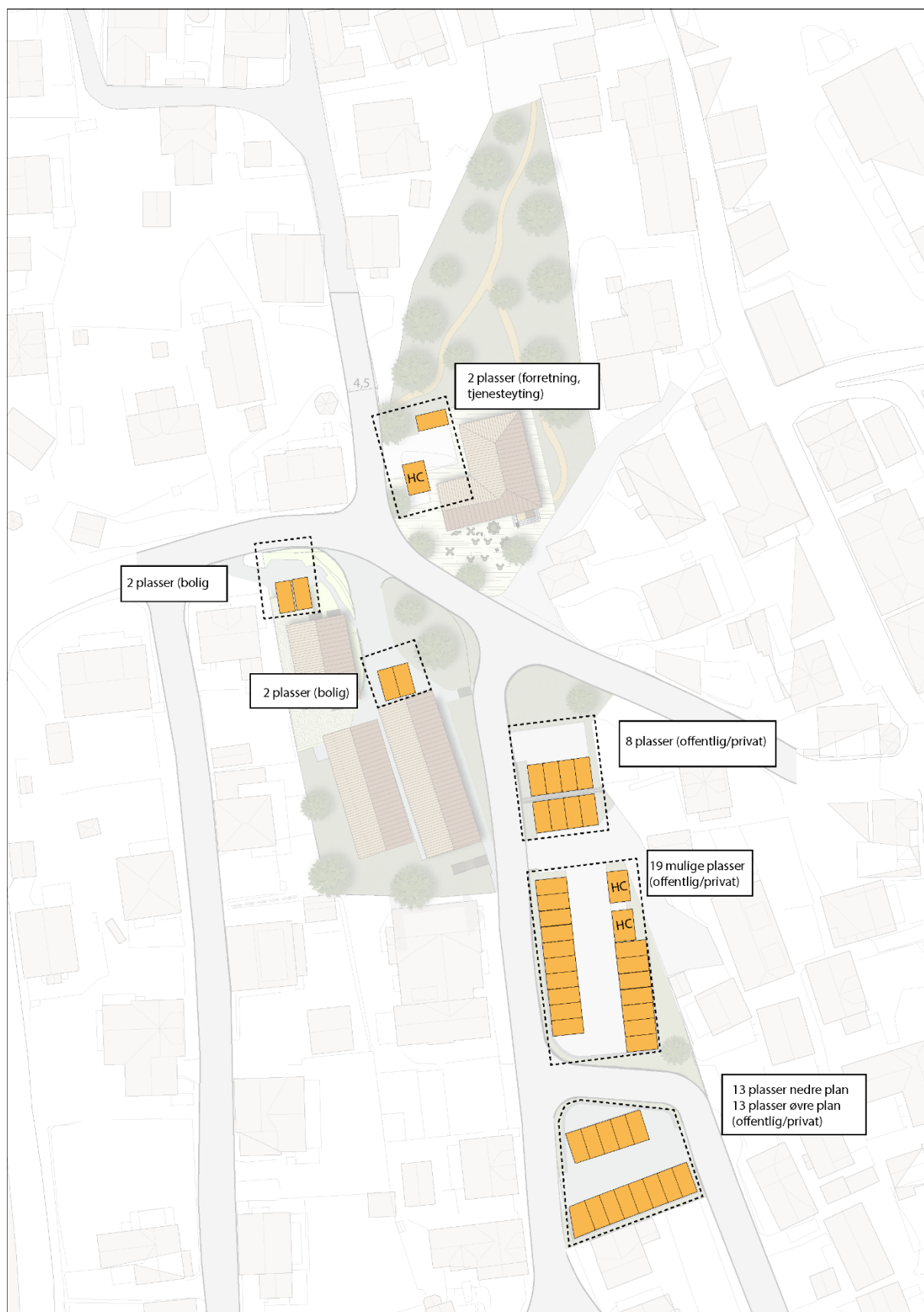
Figur 40: Forslag til situasjonsplan som viser uteareal, bebyggelse, vei og parkering.
