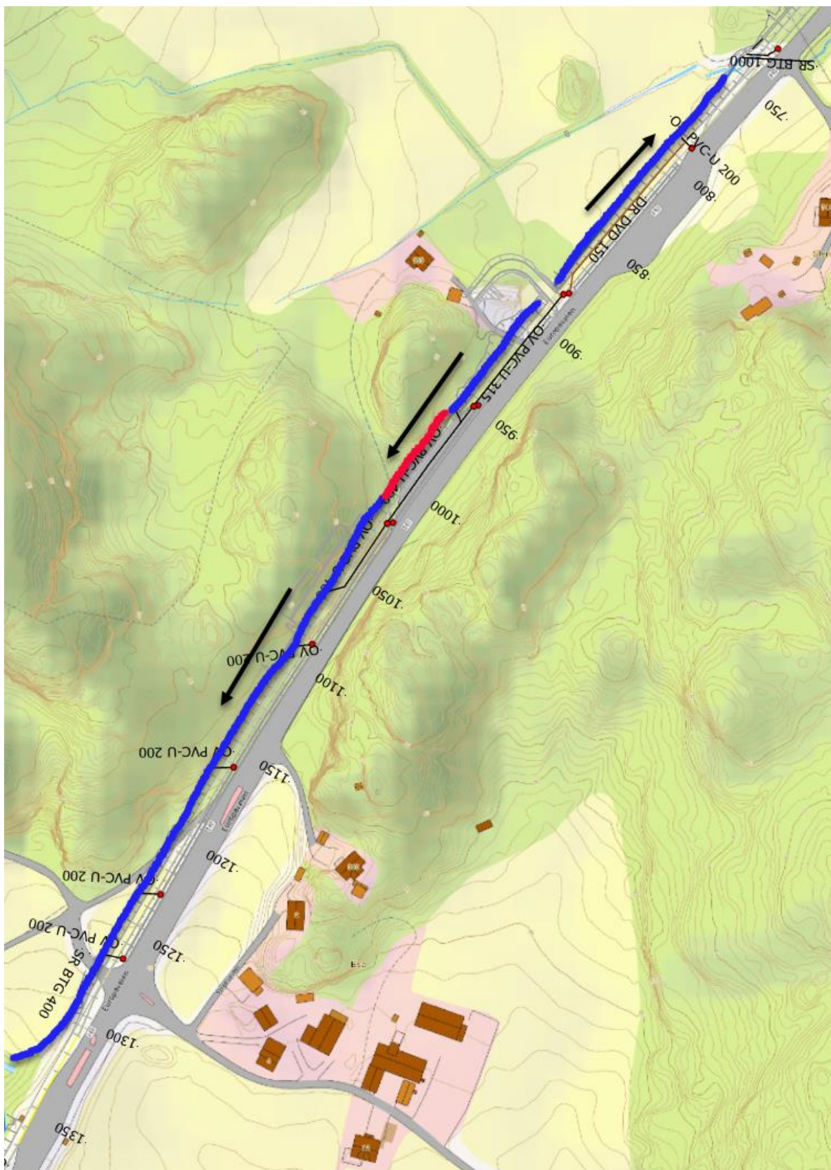
Figur 5 Hovedprinsipp for drensløsning fra P730 til P1300. Blå markering illustrerer åpen drensløsning, rød illustrerer lukket. Drensretning er markert med svarte piler.
