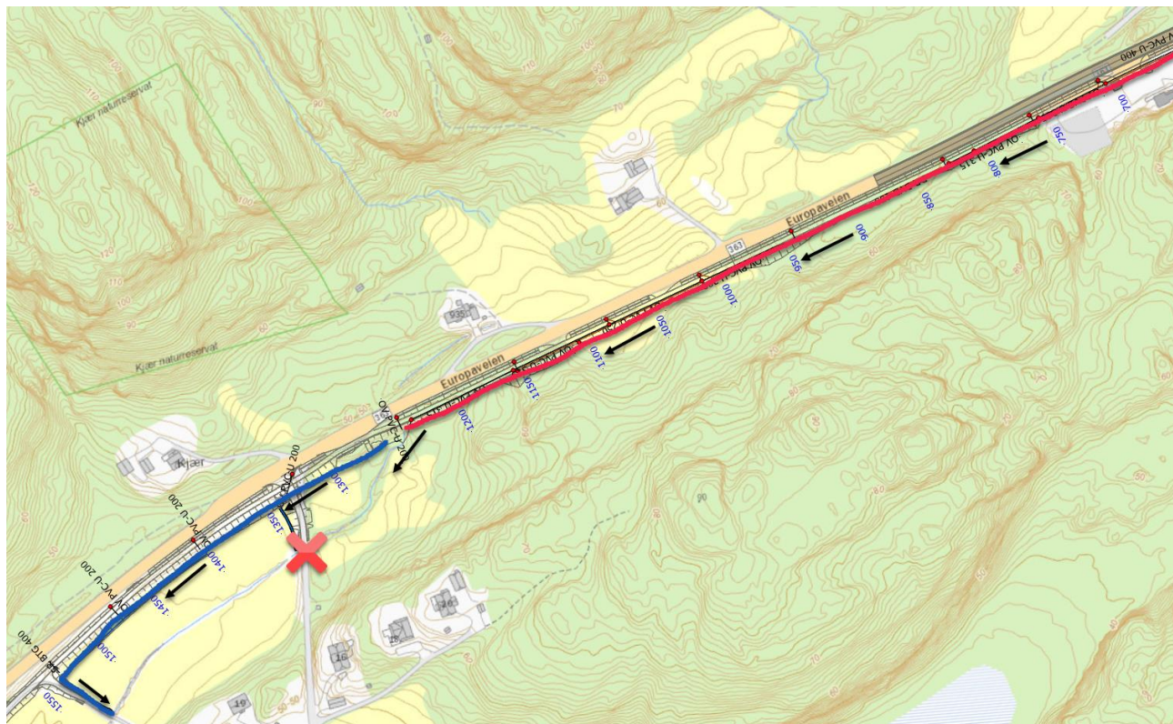
Figur 10 Hovedprinsipp for dreneringsløsning fra P700 til P1550. Blå markering illustrerer åpen dreneringsløsning, rød illustrerer lukket. Dreneringsretning er markert med svarte piler. Rødt kryss viser
