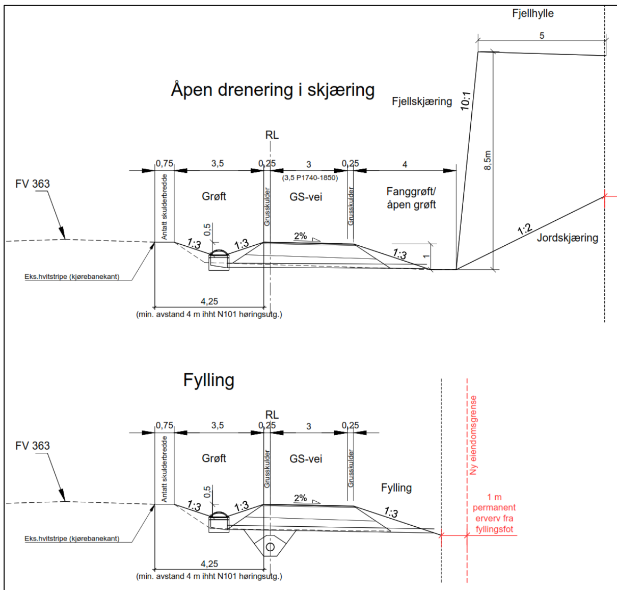
Figur 7 Normalprofil for typisk drencprinsipp for delstrekning 1 Bamble kirke - Åby
