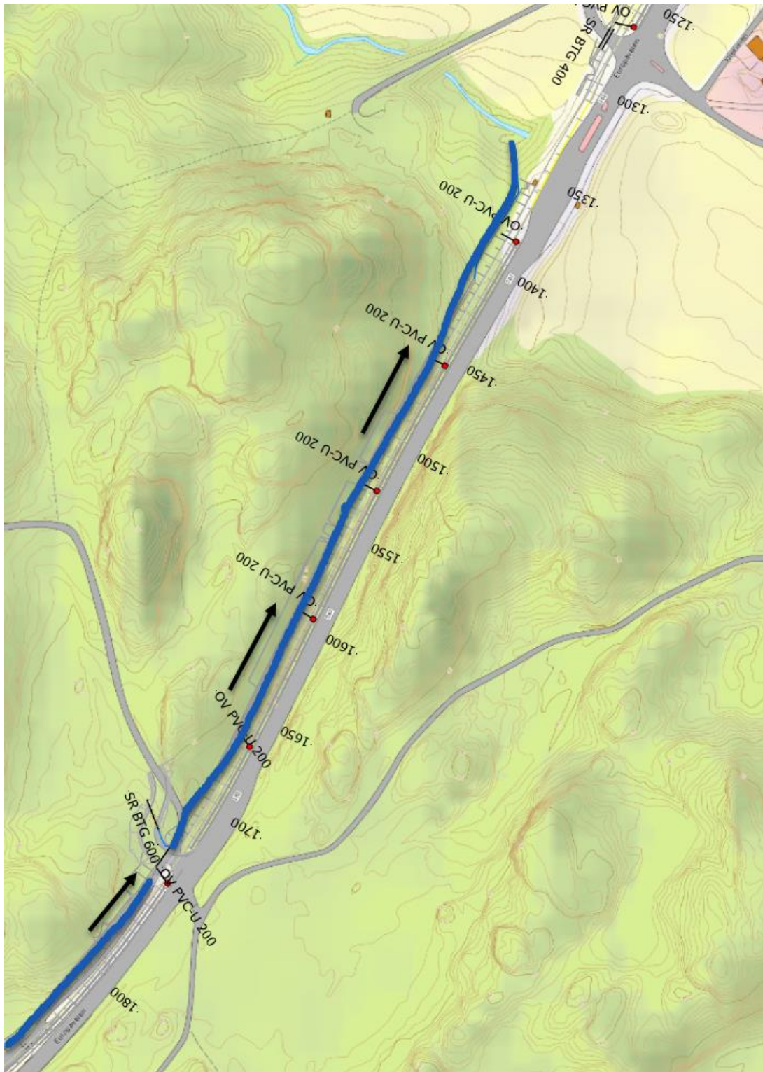
Figur 6 Hovedprinsipp for dreisløsning fra P1360 til P1780. Blå markering illustrerer åpen dreisløsning. Dreisretning er markert med svarte piler.
