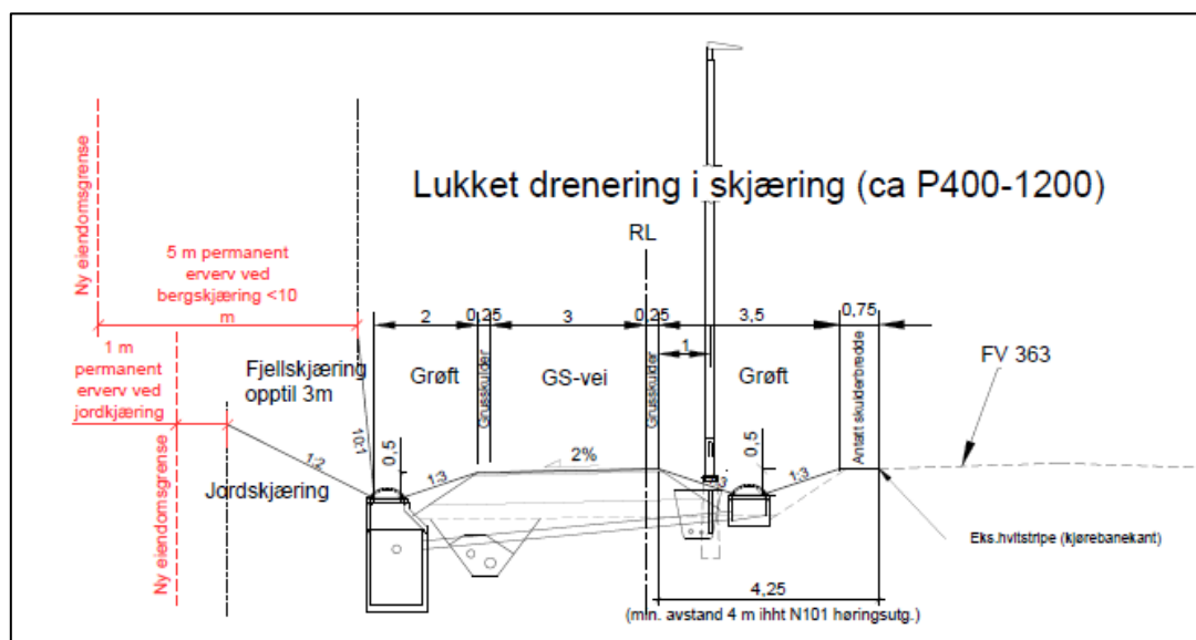
Figur 12 Typisk normalprofil for åpen løsning mellom P400-P1200. Bisluk mellom GS-veg og Fv.363 leder vann til sandfang, og videre til lukket rørgrøft.
