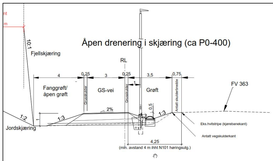
Figur 9 Typisk normalprofil for åpen løsløsning mellom P0-P400. Bisluk mellom GS-veg og Fv.363 leder vann til åpen dreneringsløsning.
