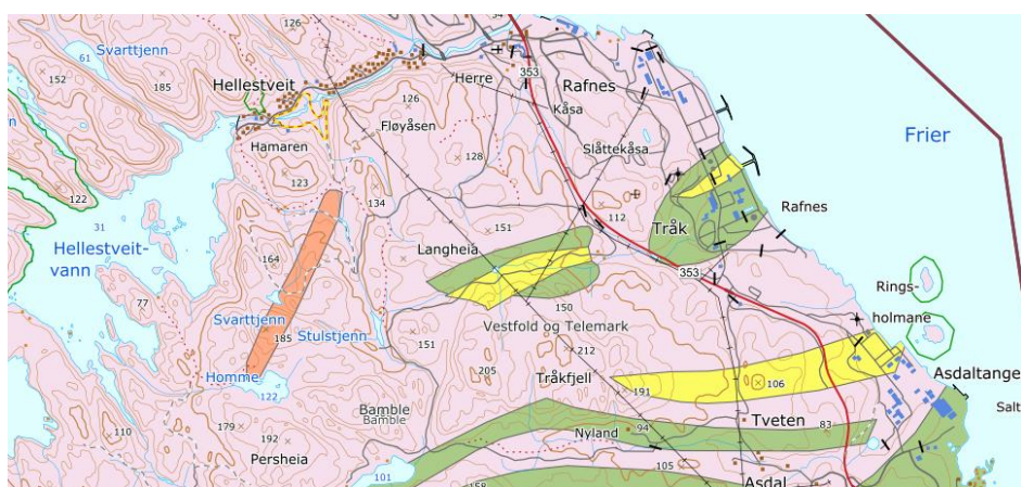
Figur 7-56 Kartutsnitt NGU Berggrunnskart 1:250.000
