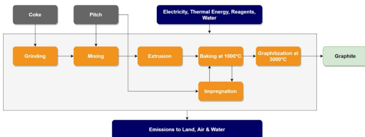
Figur 7-59 Prosessdiagram for produksjon av syntetisk grafitt. 5
