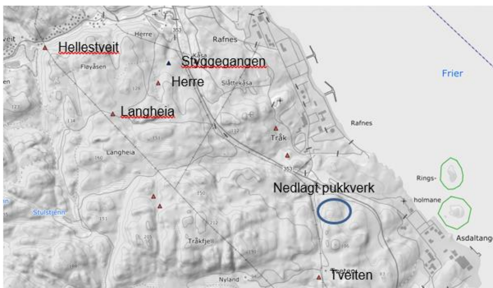
Figur 7-57 Mineralforekomster. Blå trekant=industrimetall, Rød trekant=metall. Kilde: NGU.no
