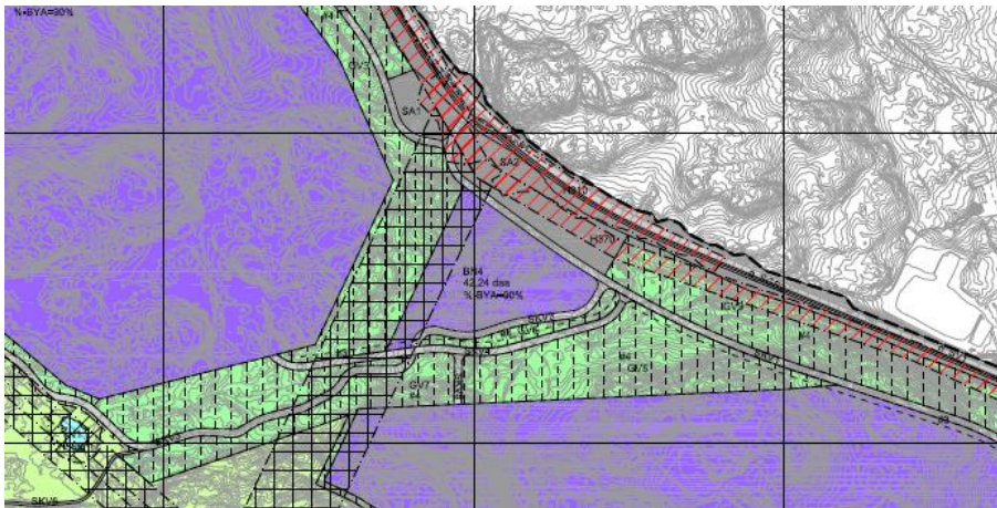
Figur 4-9 Utsnitt reguleringsplan BN4
