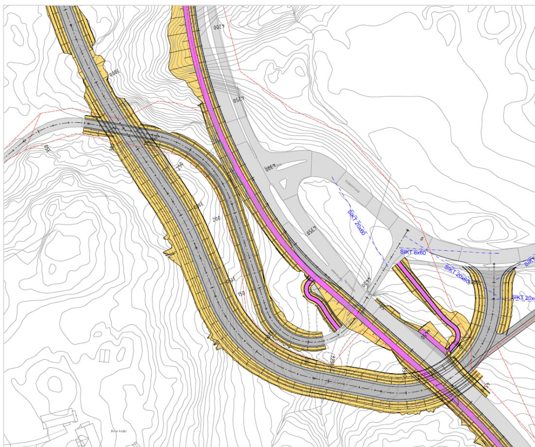
Figur 4-13 Skisse nytt kryss i sør
