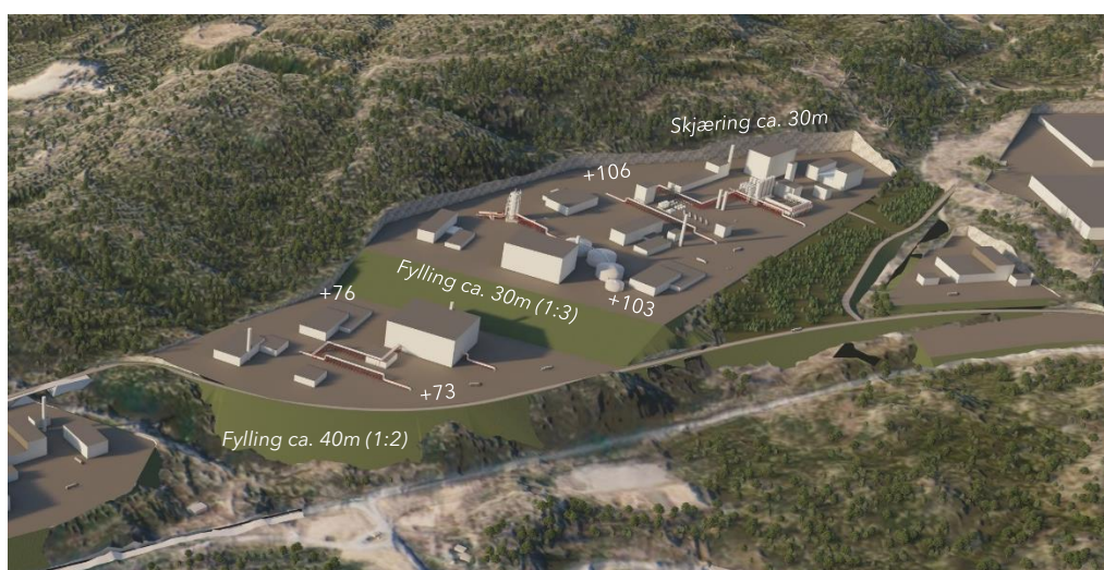
Figur 4-6 Illustrasjonsplan BN2 3D-modell med kotehøyder på flatene
